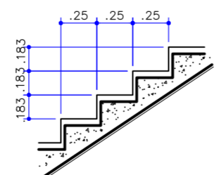
DET. DEGRAUS ESCALADA INTERNA SEM ESCALA
