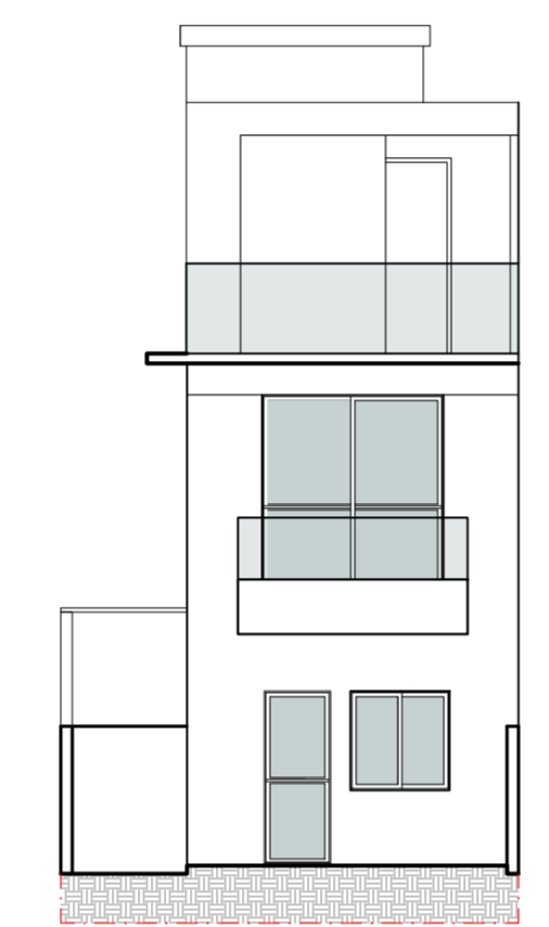
CASA TIPO B1 ESQUERDA ELEVÇÃO FRONTAL ESC. 1:100
