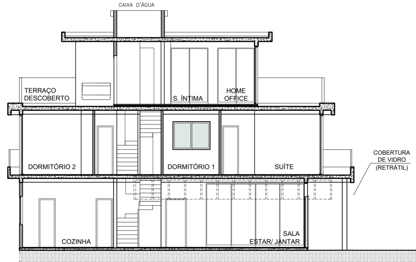
CASA TIPO B1 ESQUERDA CORTE AA ESC. 1:100
