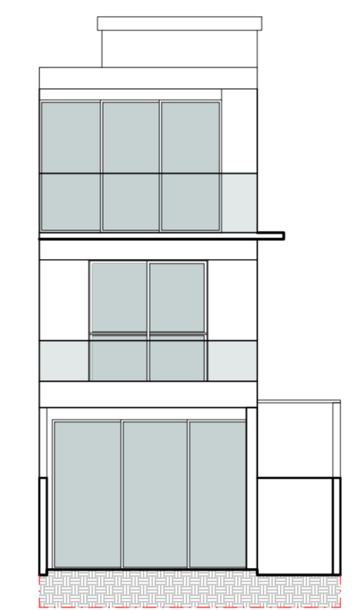
CASA TIPO B1 ESQUERDA ELEVÇÃO POSTERIOR ESC. 1:100
